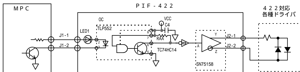
【回路図】
